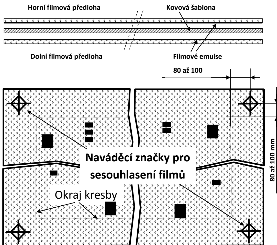
Provedení filmových předloh pro výrobu leptané šablony
